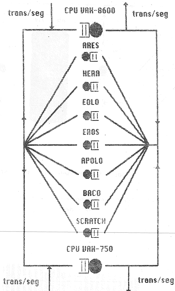
FIGURA 3.1 - Modelo abierto sistema UAH-8600/UAH-750
